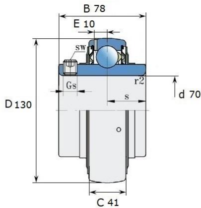
Размеры (мм): LE 314 2F
