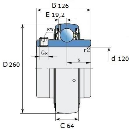
Размеры (мм): LE 324 2F
