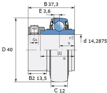
Размеры (мм): LY 202-009 2F
