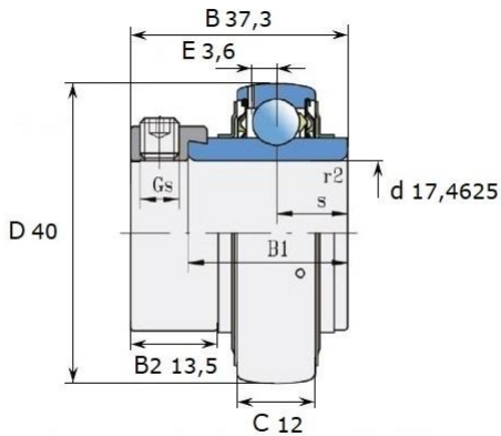
Размеры (мм): LY 203-011 2F
