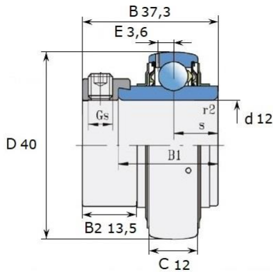
Размеры (мм): LY 203/12 2F
