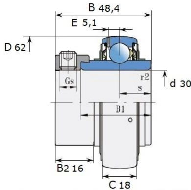
Размеры (мм): LY206-2F
