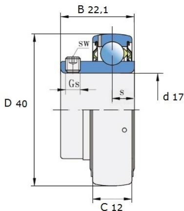
Размеры (мм): UE 203-2S
