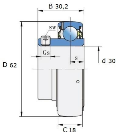
Размеры (мм): UE 206-2S
