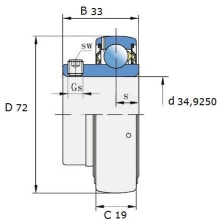
Размеры (мм): UE 207-106 2S
