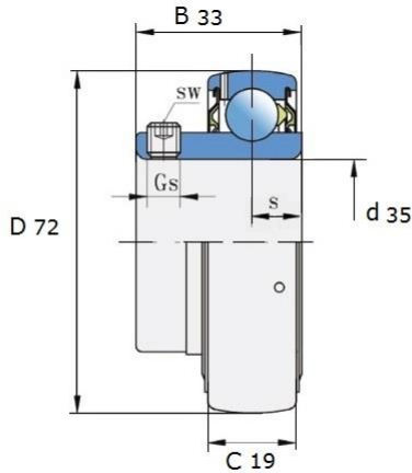
Размеры (мм): UE 207 2S
