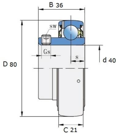
Размеры (мм): UE 208 2S
