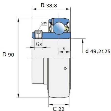
Размеры (мм): UE 210-115 2S
