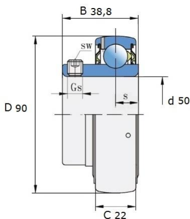
Размеры (мм): UE 210-2S
