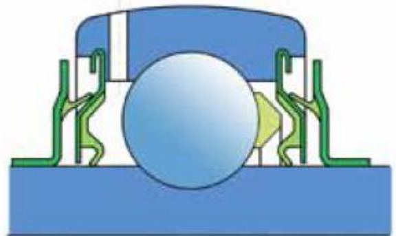
Уплотнение 2В
