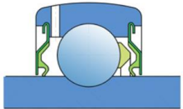
Уплотнение 2RS
